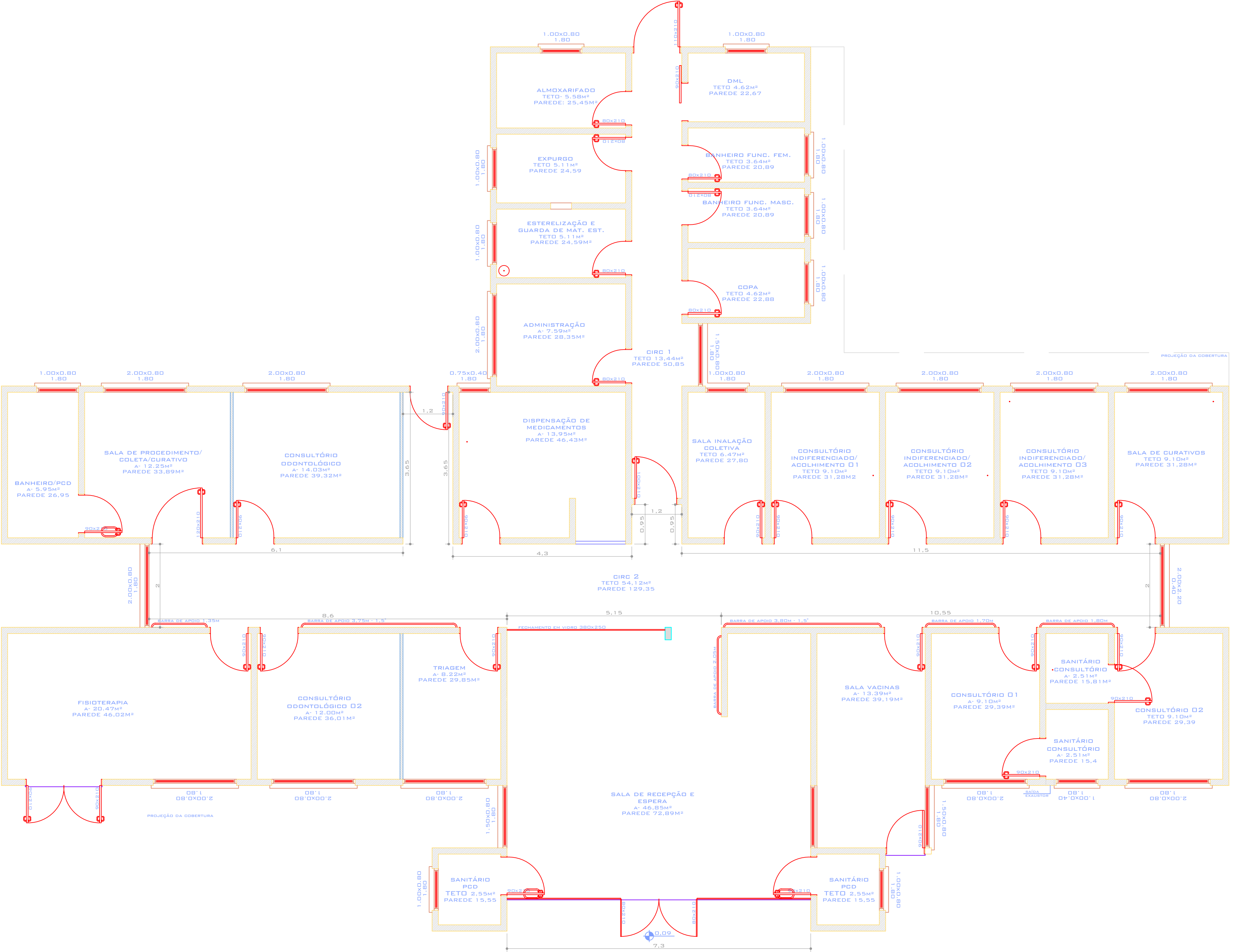
PLANTA BAIXATERREO
